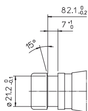
ISO 40 OTT
