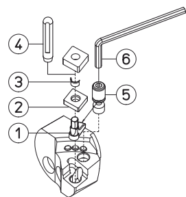
PCLNR/L
